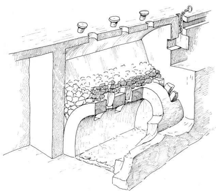
Rekonstruktion der indirekten Heizungsanlage im Augustinerkloster (nach Palmowski 1986). Rechteinhaber: TLDA Weimar
