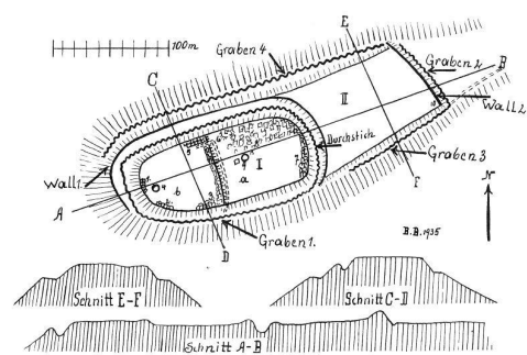
Die Burganlage auf dem Hausberg von Langenberg. Plan nach Brause 1934. Rechteinhaber: TLDA Weimar
